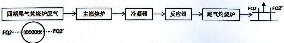
图 3 有组织废气采样示意图
