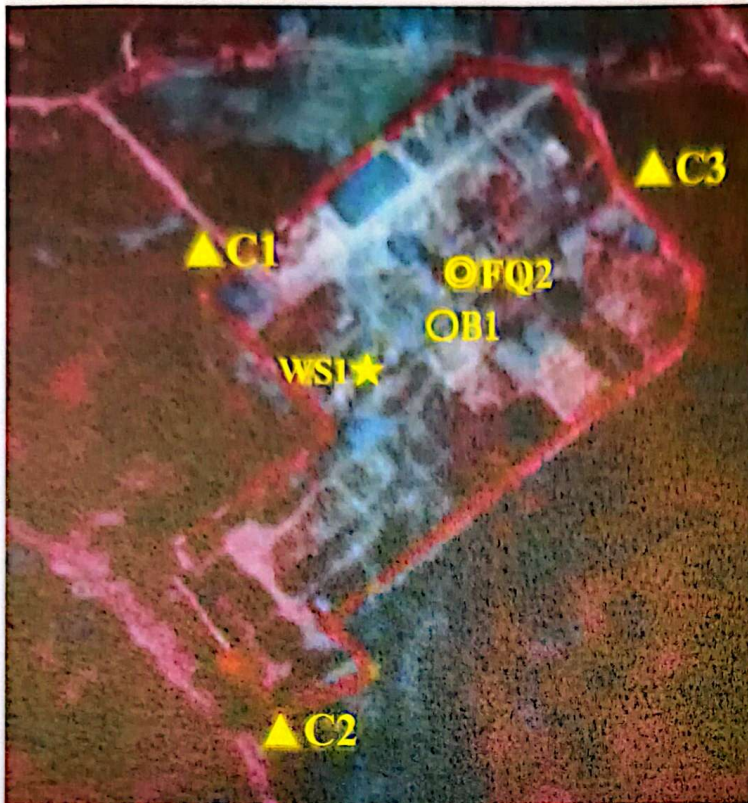
图 1 废水、有组织废气、无组织废气和厂界噪声监测布点示意图
