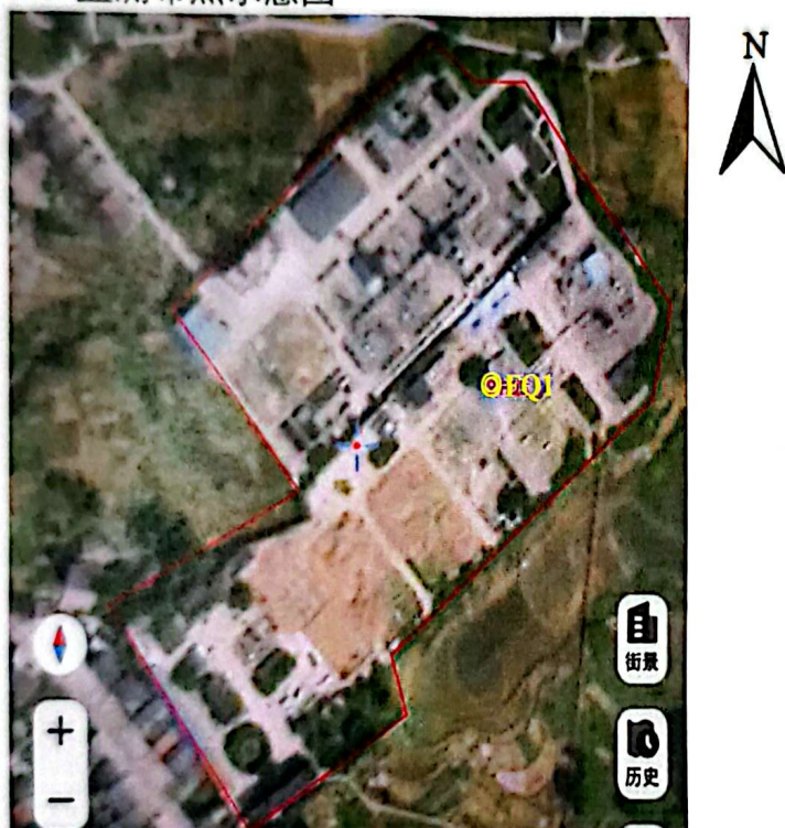
图 1 有组织废气监测布点示意图
