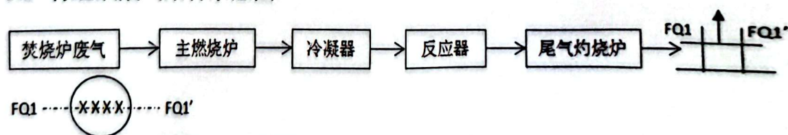
图 2 有组织废气采样示意图
